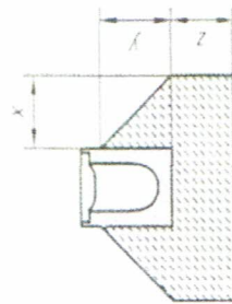
Rys. 1. Wymiary podparcia.
