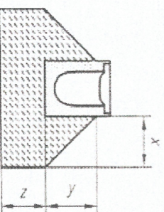
Rys. 1. Wymiary podparcia.
