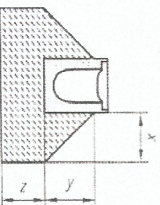
Rys. 1. Wymiary podparcia.
