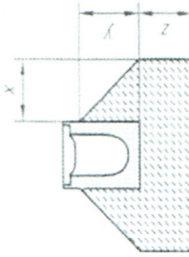
Rys. 1. Wymiary podparcia.
