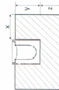
Rys. 1. Wymiary podparcia.
