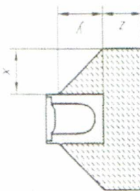
Rys. 1. Wymiary podparcia.
